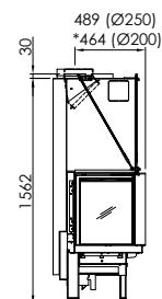
Linear Corner 46x46x57 (P. 38) Mini 2LRh-57-4S
